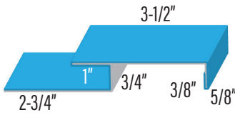
BATTEN TRIM PROBOARD PBBT
