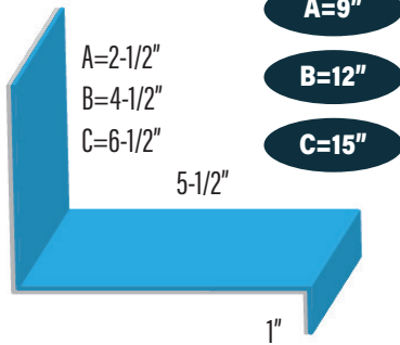
SKYLITE 2-A, B, C PROLOK PRSKY2-A,B,C
