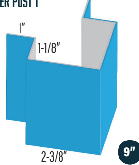
DURACLAD/ALLCLAD/DIAMOND DCOCP
