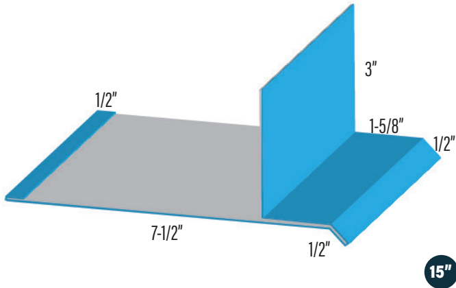
DOOR MOLDING DRIP DMD1
