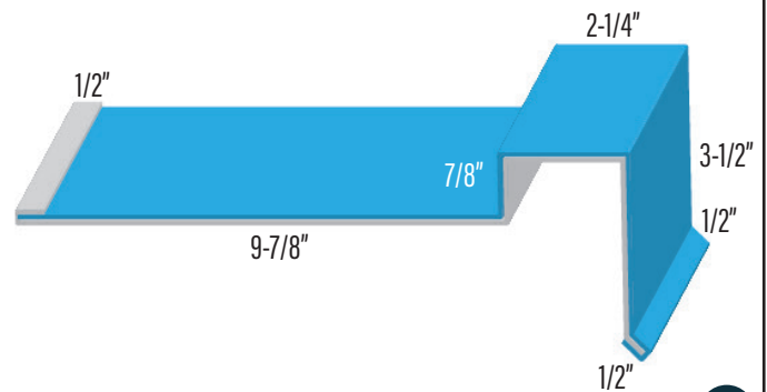
DURACLAD/ALLCLAD/DIAMOND DCPROW
