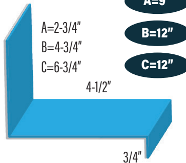
SKYLITE 2-A, B, C DURACLAD/ALLCLAD/DIAMOND DCSKY2-A,B,C
