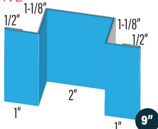
SOFFIT DRIP WF-HF SODC
