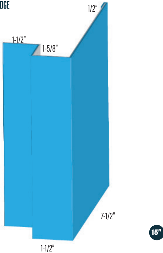
DOOR MOLDING EDGE DM2
