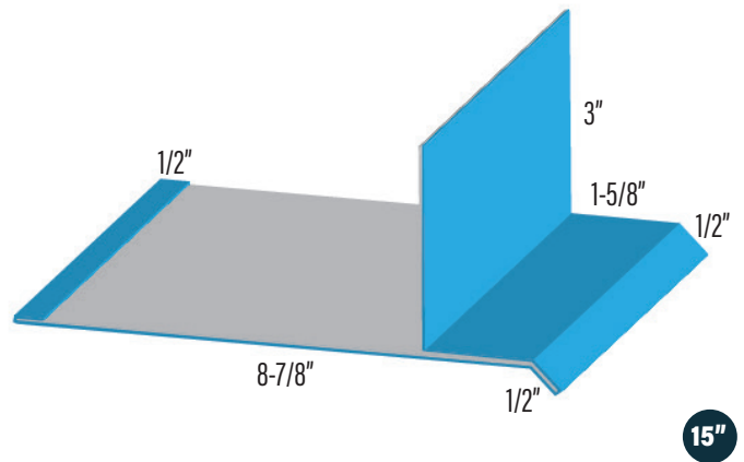
DOOR MOLDING DRIP DMD2
