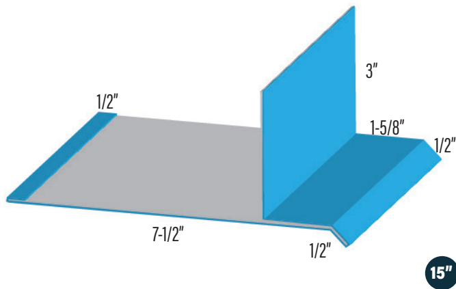
DOOR MOLDING DRIP DMD1
