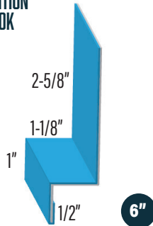
STARTER BOX DURACLAD/ALLCLAD/ DIAMOND SB1
