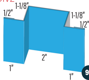
SOFFIT DRIP WF-HF SODC
