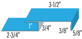
BATTEN TRIM PROBOARD PBBT
