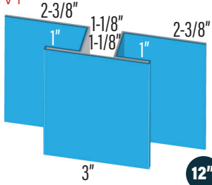
BATTEN TRIM PROBOARD PBBT
