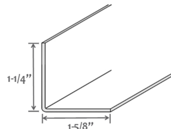
L-Trim
