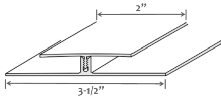
Clipsable H-Trim
