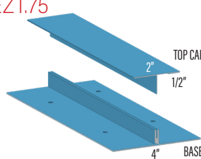
O/S CORNER QLOC.75
