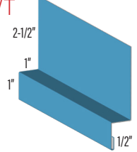
I/S CORNER QLIC.75
