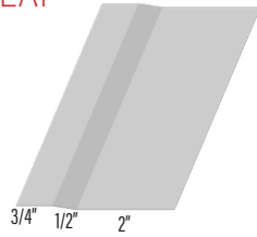
J TRIM 2 DCJT2
