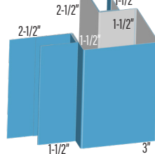
O/S CORNER QLOC1
