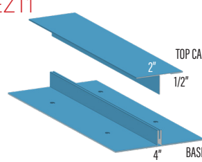
O/S CORNER QLOC1
